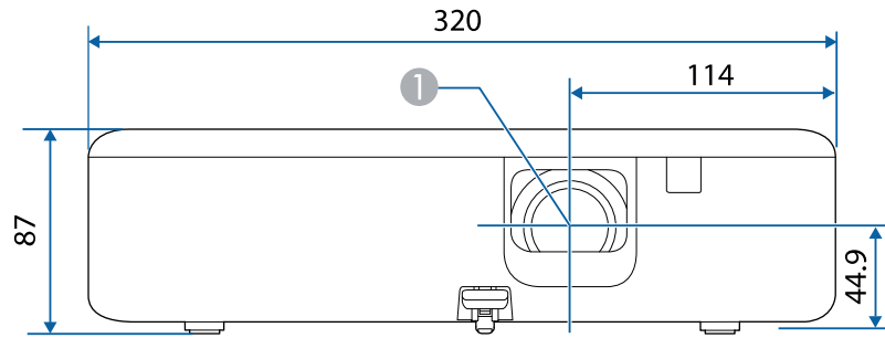
① Linssin keskikohta
